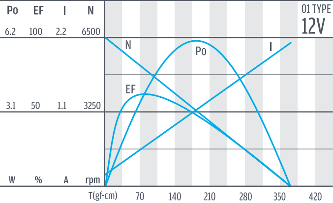
馬達單體特性/ Motor Characteristics
