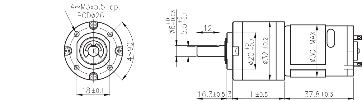
外形尺寸/ Appearance Size
