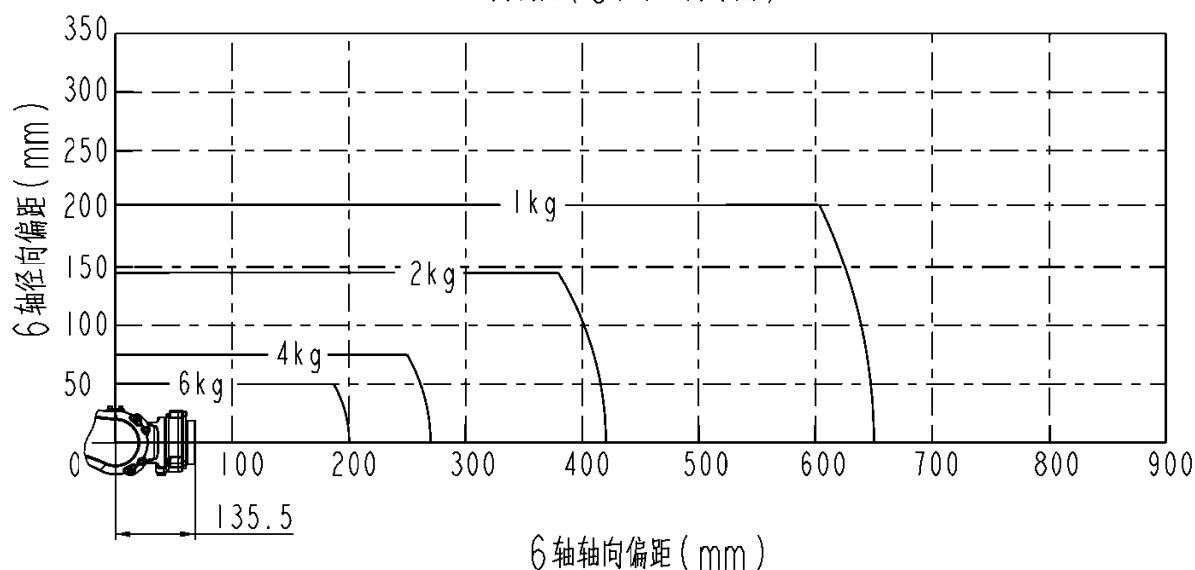
负载图 (5 轴中心为零点)
