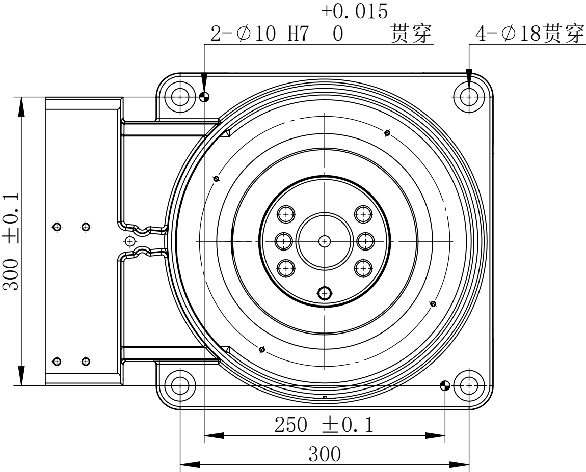
底座安装图
