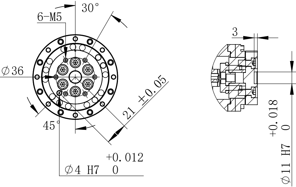
法兰安装图
