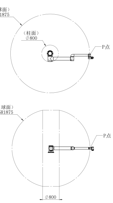
AUBO-iS20L Pro 本体P点运动范围
