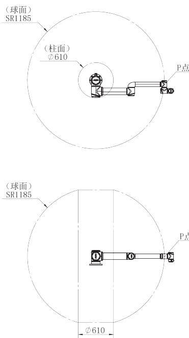
AUBO-iS10 Pro 本体P点运动范围
