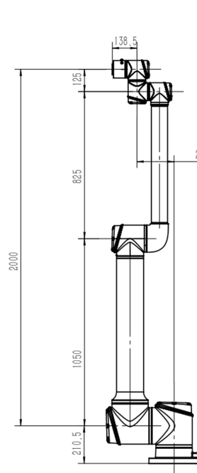
AUBO-iS20L Pro 外形尺寸图
