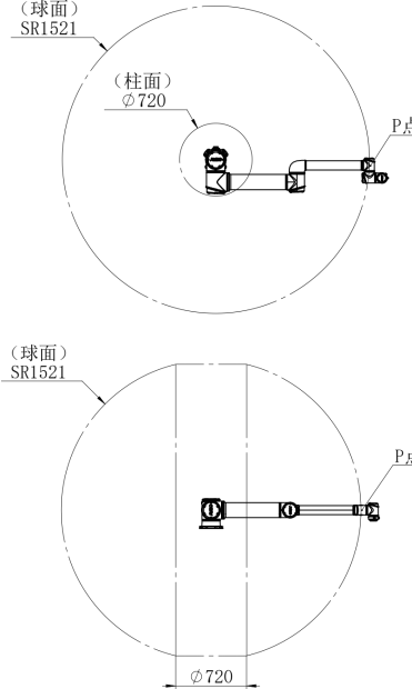
AUBO-iS20 Pro 本体P点运动范围
