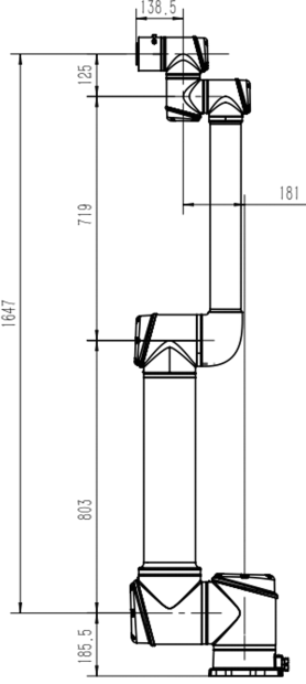
AUBO-iS20 Pro 外形尺寸图
