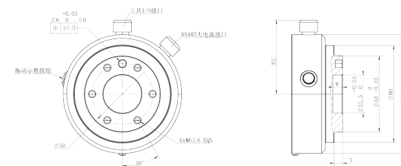
AUBO-iS25 末端法兰
