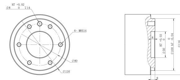
AUBO-iS35 末端法兰
