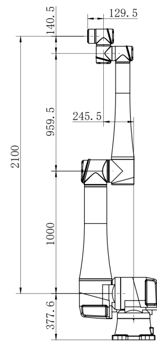
AUBO-iS35 外形尺寸图
