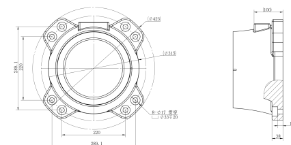
AUBO-iS35 基座图
