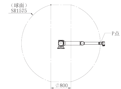
AUBO-iS25 本体P点运动范围
