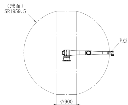
AUBO-iS35 本体P点运动范围
