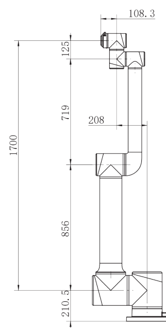
AUBO-iS25 外形尺寸图
