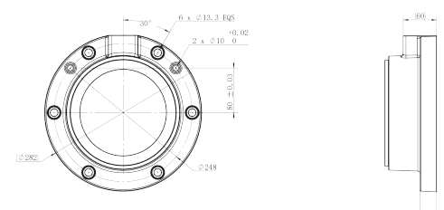
AUBO-iS25 基座图
