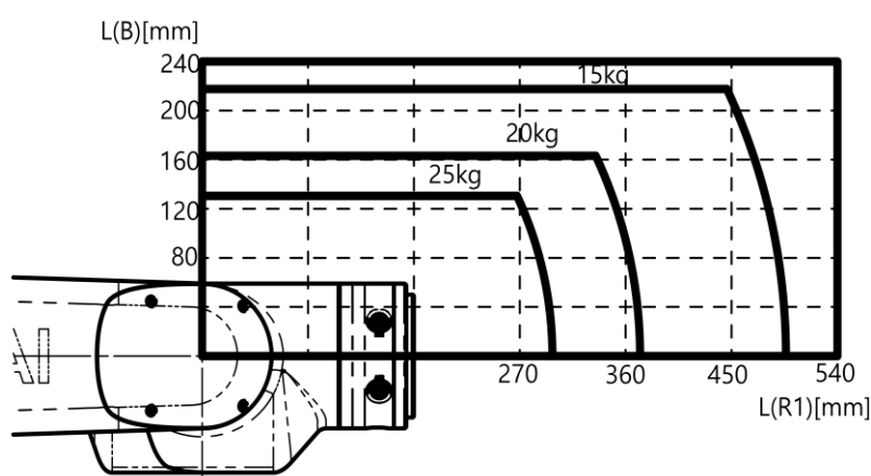
손목축 토크 선도
