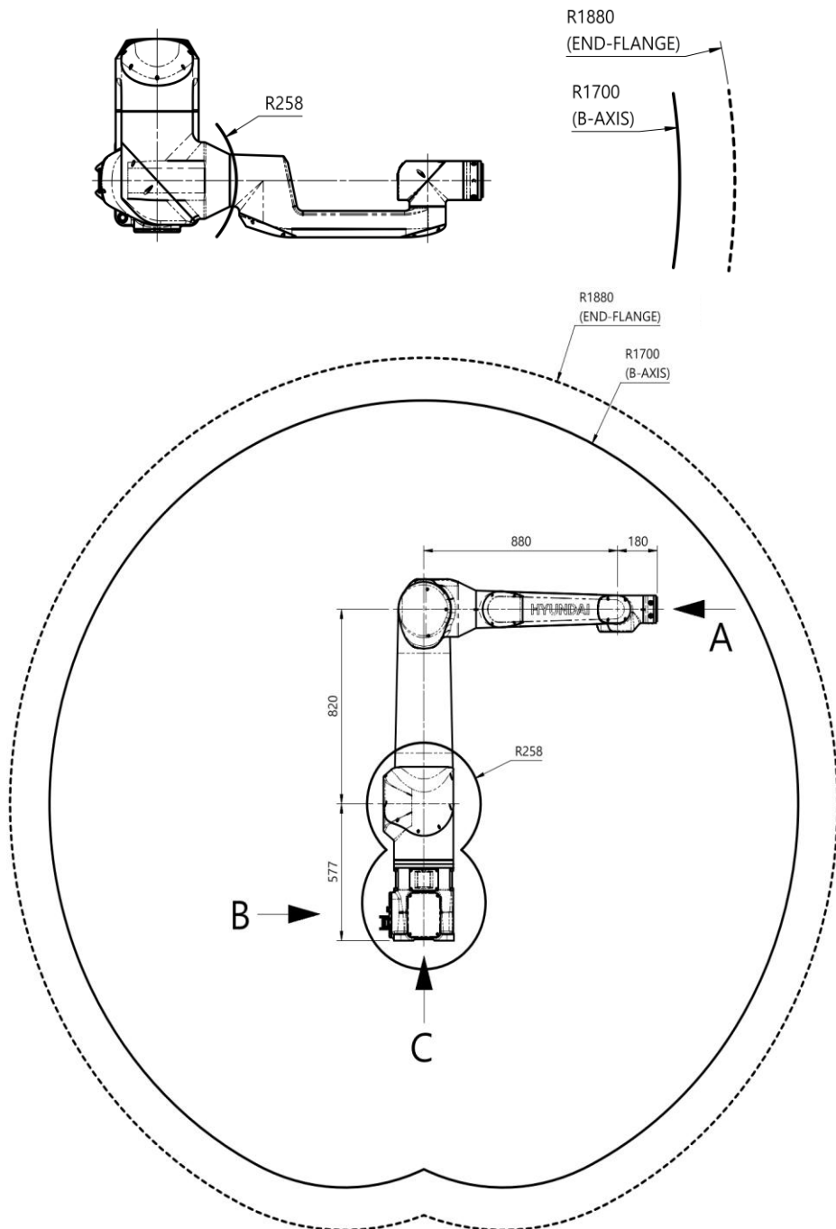
VIEW A 손목 취부부 상세도
