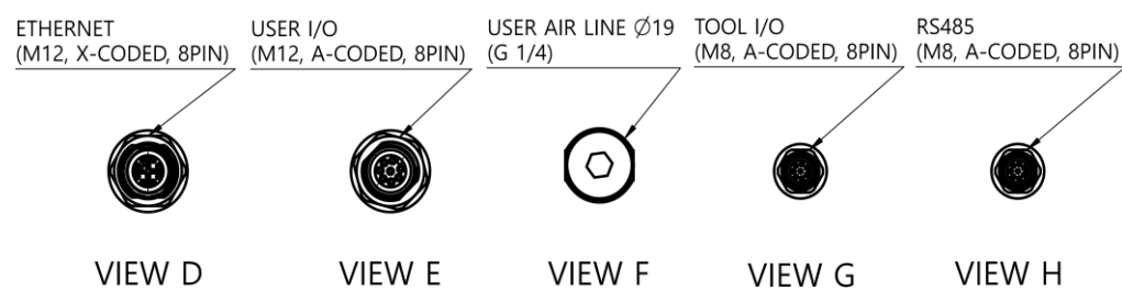
VIEW D, E, F, G, H 응용 케이블 접속부
