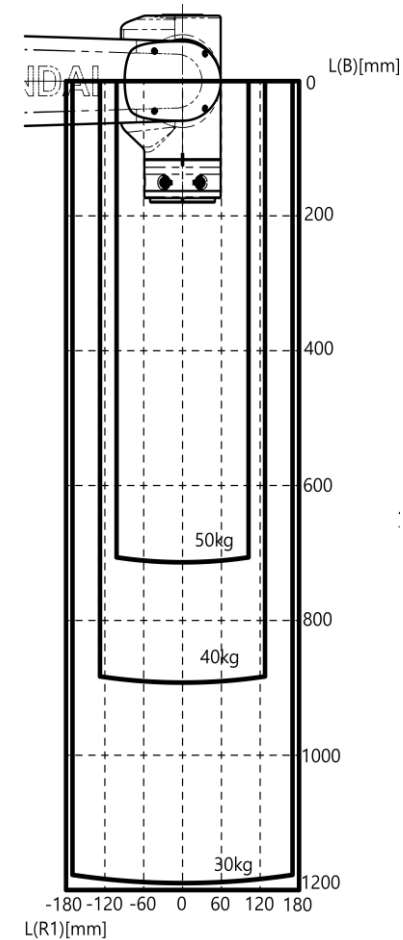
손목축 토크 선도
