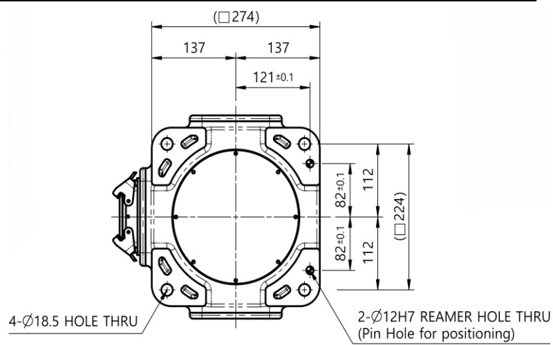
VIEW D, E, F, G, H 응용 케이블 접속부
