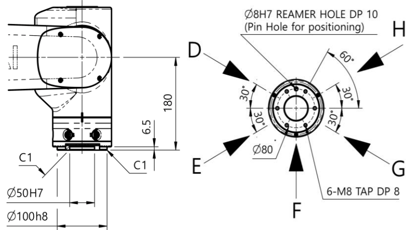
VIEW C 본체 바닥설치 치수도
