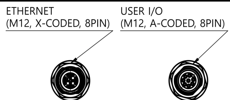
VIEW D, E 응용 케이블 접속부
