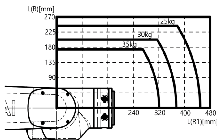
손목축 토크 선도
