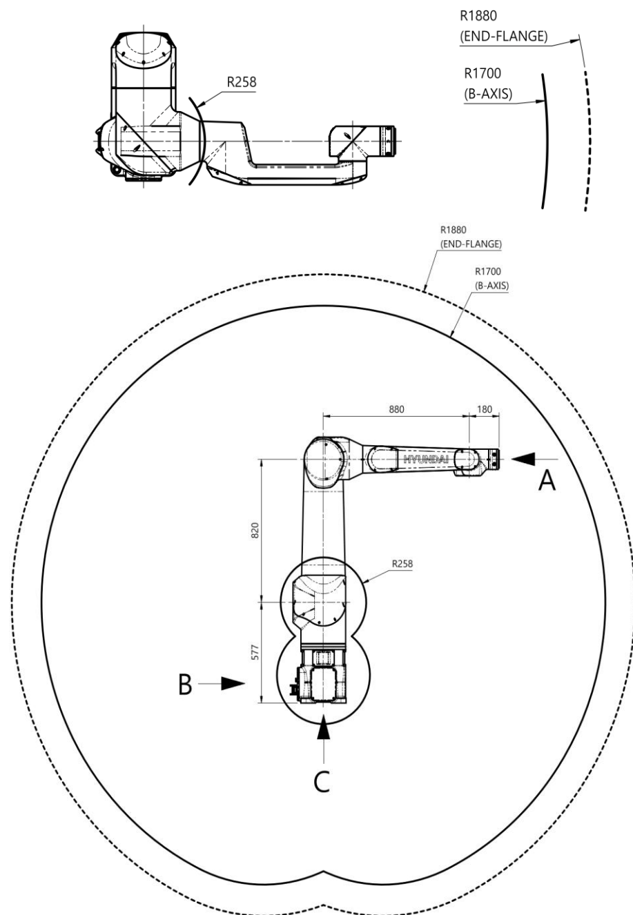
VIEW A 손목 취부부 상세도
