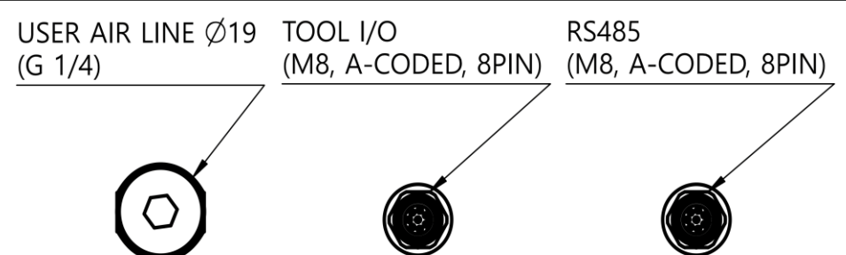
VIEW F, G, H 응용 케이블 접속부
