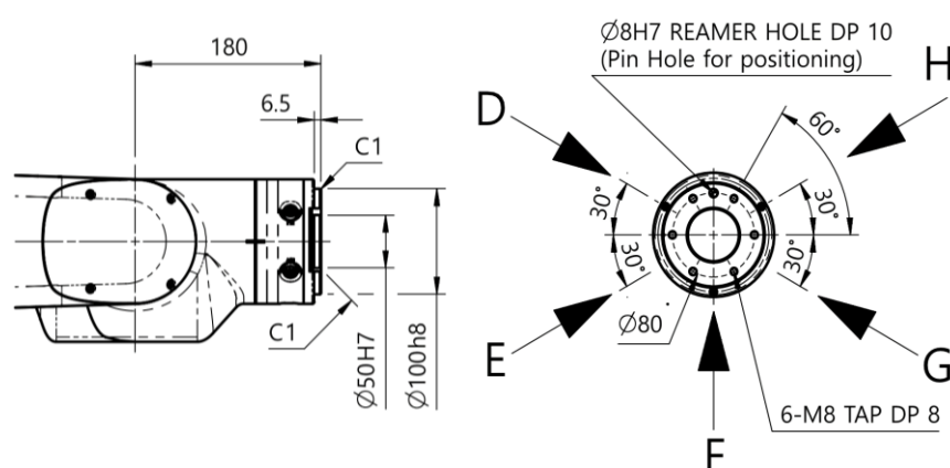
VIEW C 본체 바닥설치 치수도
