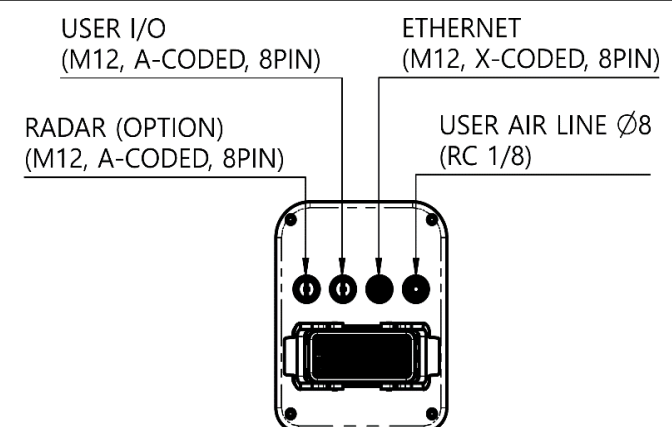
VIEW D, E 응용 케이블 접속부
